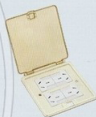
DHM-628/GU / 铜合金 Copper alloy 126×120mm
