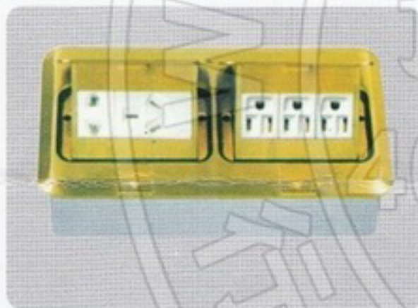
JLT-200F 单相二、二极插座10A 250A、三位电脑电源插座
