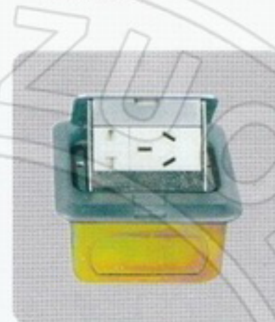
型号: JLT-120F1 规格: 一位二极插座 一位三极插座
