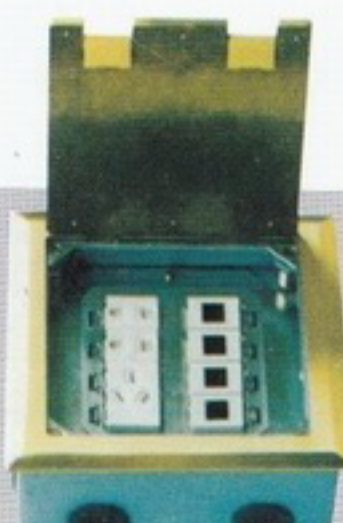
JLT-180K 二位二极双用插座、一位二极带接地插座 四位安普电脑插座（模块另配）
