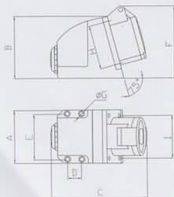
尺寸简图 DIMENSIONS CHART
