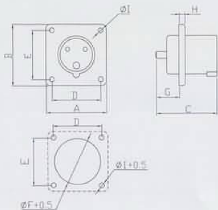
尺寸简图 DIMENSIONS CHART
