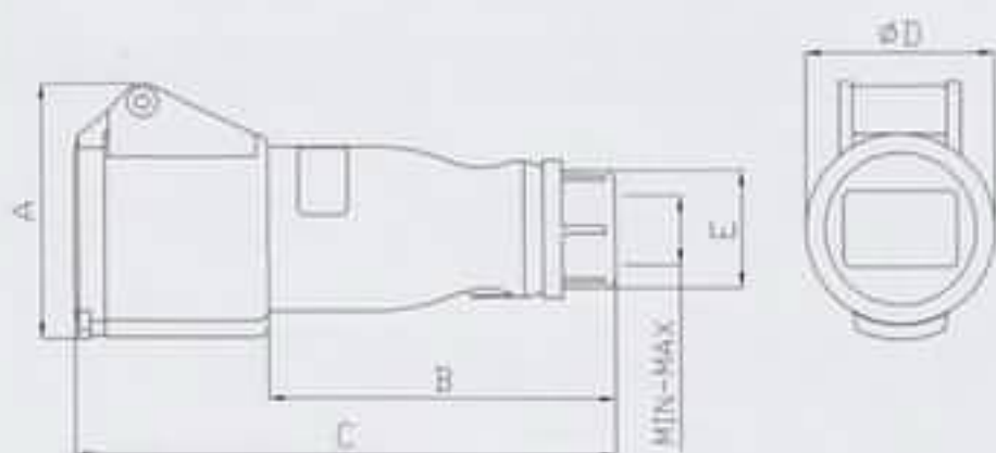
尺寸简图 DIMENSIONS CHART
