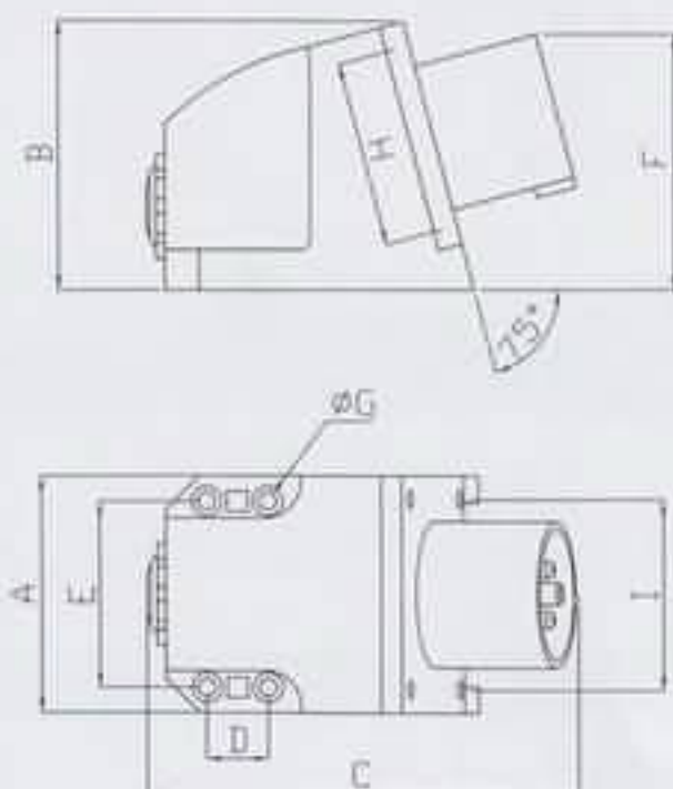
尺寸简图 DIMENSIONS CHART
