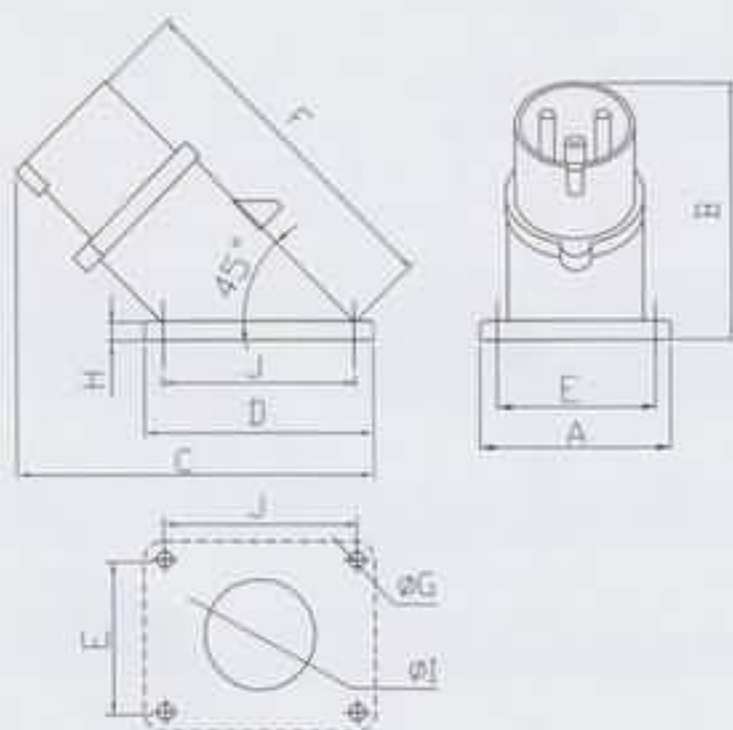
尺寸简图 DIMENSIONS CHART
