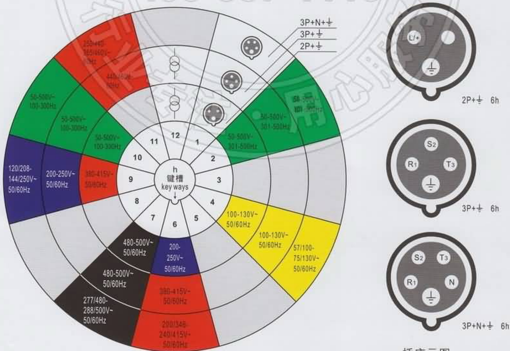
插座示图
